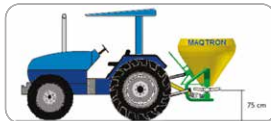
O distribuidor é acoplado diretamente no 3º ponto do hidráulico do trator.
