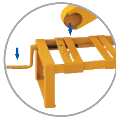
Base com esticador (para motor elétrico e à combustão) Correia ind. 2un.VA 49 a 55 ref. mod. M-613
